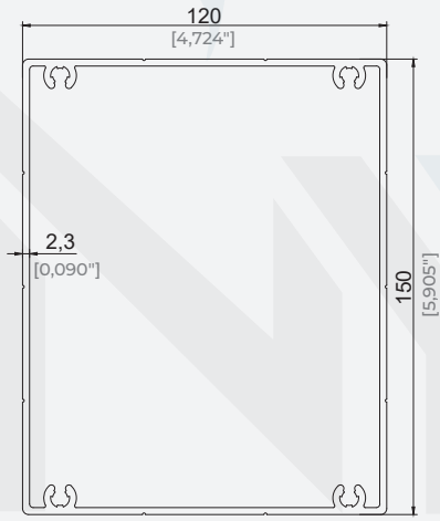
120x150 Dikme Profili 120x150 Pillar Profile
