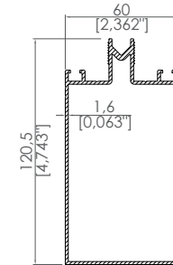
Standart Cam Taşıyıcı Standart Glass Carrier Profile
