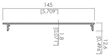
Motor Kutusu Kapak Profili Motor Box Cover Profile
