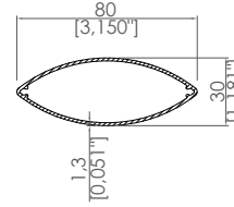
80x30 Güneş Kırıcı Profili 80x30 Sun Breaker Profile
