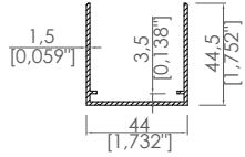
Panel Dikme Bağlantı Profili Panel - Pillar Connection
