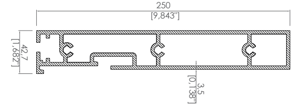
Yan Kayıt Profili Side Beam Profile
