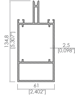
61x134,8 Cam Taşıyıcı 61x134,8 Glass Carrier Profile
