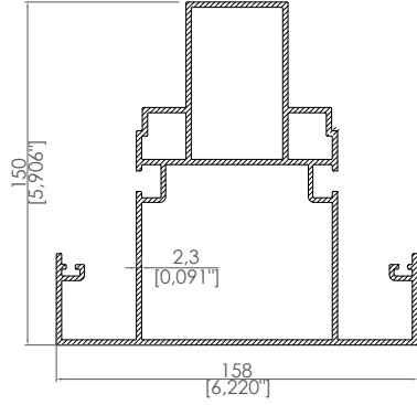
Orta Taşıyıcı Profili Middle Beam Profile
