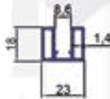
Cod: 2150 - 0,375 kg/m 8 mm Cam Adaptör Profili
