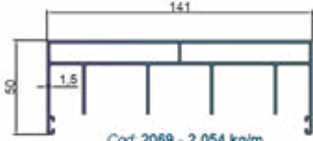
Cod: 2069 - 2,054 kg/m Üst Kasa Profili
