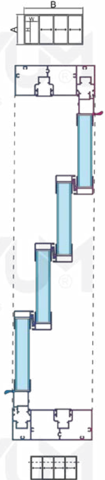
DÖRTLÜ SİSTEM QUATERNARY SYSTEM
