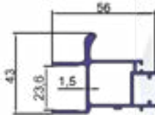
Cod: 2068 - 0,878 kg/m Kulplu Yan Çerçeve Profili
