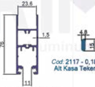
Cod: 2565 - 1,205 kg/m Alt Çerçeve Profili
