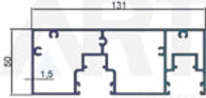
Cod: 2066 - 2,414 kg/m Yan Kasa Profili
