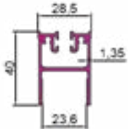
Cod: 2071 - 0,703 kg/m Üst Çerçeve Profili
