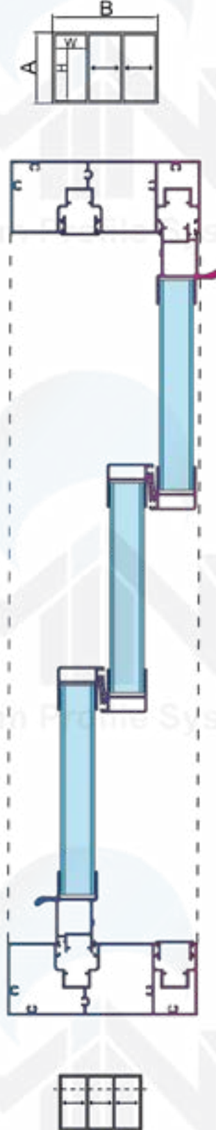
ÜÇLÜ SİSTEM TRIPLE SYSTEM
