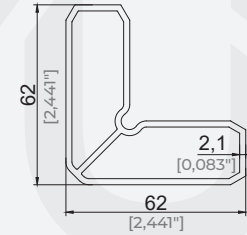
KASA KÖŞE TAKOĞU PROFİLİ FRAME CORNER WEDGE PROFILE
